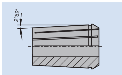
Collet taper angle 2°52': DIN ISO 10897. Collet taper angle 8°: DIN ISO 15488.
