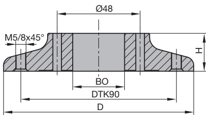
Flange TR 810 0
