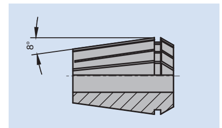
Collet taper angle 2°52': DIN ISO 10897. Collet taper angle 8°: DIN ISO 15488.
