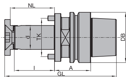
Arbor HSK-E 63
