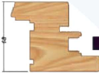
0900-12 HM Z: 3+3 D: Ø160 d: Ø35
