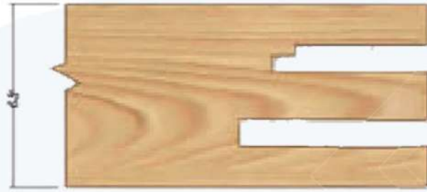
0900-04 HM Z: 4 D: Ø270 d: Ø35
